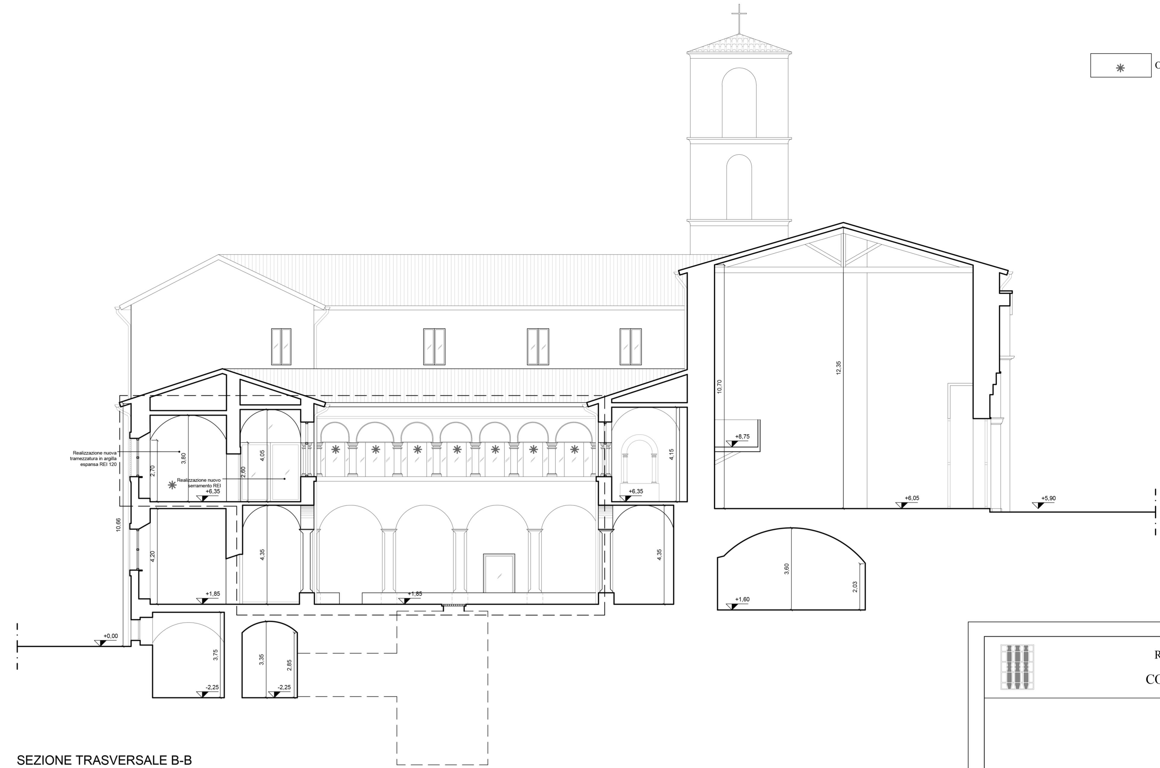
SEZIONE TRASVERSALE B-B
